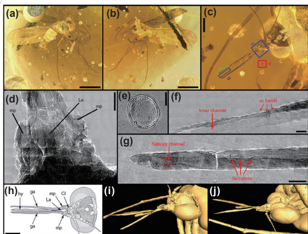
◎ Parapolycentropus parabormiticus 頭部與花粉的穿透式 X 光顯微鏡 (TXM) 與微米 X 光斷層掃描重建影像，其中 (a) 為右視圖、(b) 為左視圖、(c) 為上視圖、(d) 為長鼻基部的 TXM 影像、(e) 為 (c) 中的紅色方框放大的花粉 TXM 影像、(f) 為 (c) 中綠色方框口器尖端的 TXM 影像、(g) 為 (c) 黑色方框中下頷骨尖端和相關外部裝飾物的 TXM 影像、(h) 為 (c) 中的頭部和長鼻示意圖、(i) 與 (j) 為微米 X 光斷層掃描頭部的 3D 重建。(a) 和 (b) 中比例尺代表 1 mm；(c) 和 (h) 為 0.2 mm；(d) 中為 30 \mu m；(e) 中為 10 \mu m；(f) 中為 15 \mu m；(g) 中為 20 \mu m。
